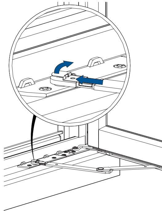
Drehbegrenzer aushängen
