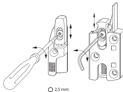
Rahmenteil DFE/TFE
